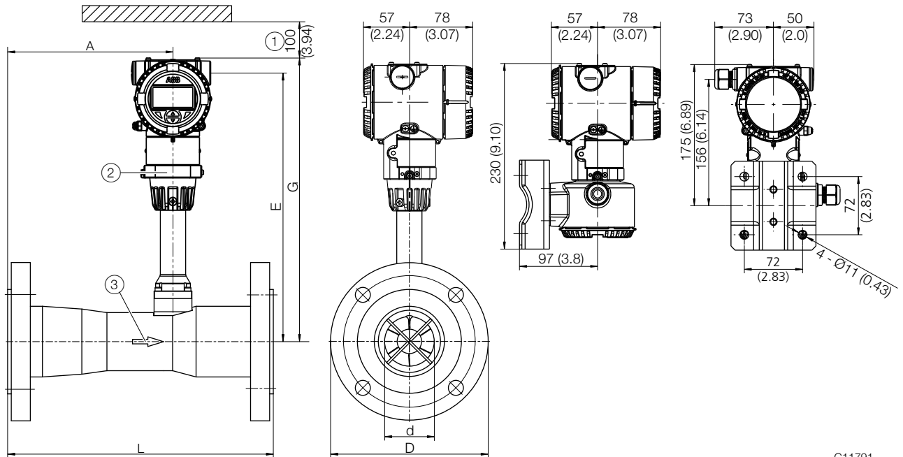
Рис. 13: Размеры в мм (inch)
