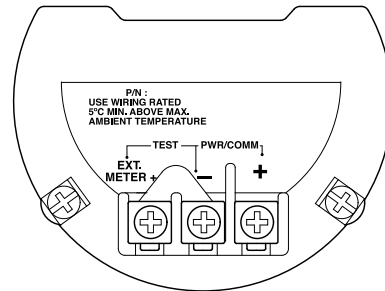
Рис. 14: Соединительные клеммы
