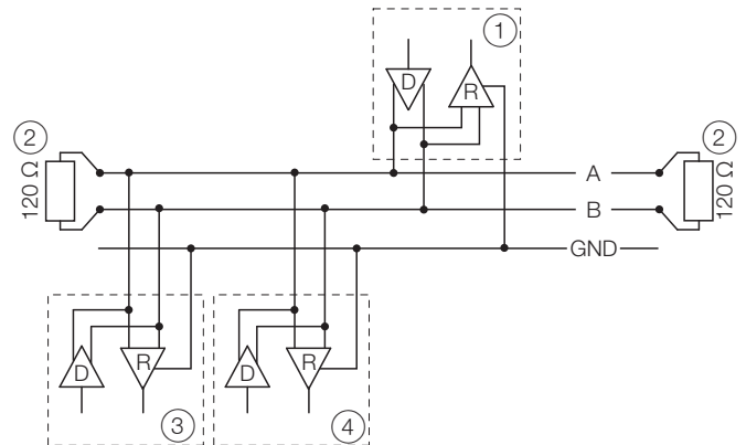
Рис. 18: сеть Modbus (пример)
