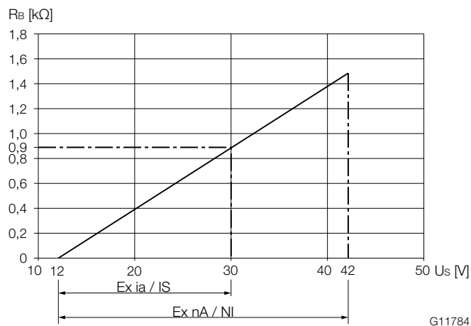
Рис. 26: питание в зоне 0, 1, 2, взрывозащита «Искробезопасность / Intrinsically safe»
