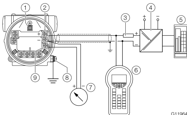
Рис. 16: Связь по протоколу HART (пример)
