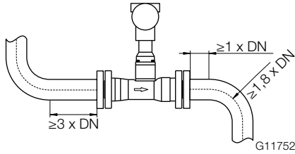
Рис. 8. Участки трубопровода с коленом
