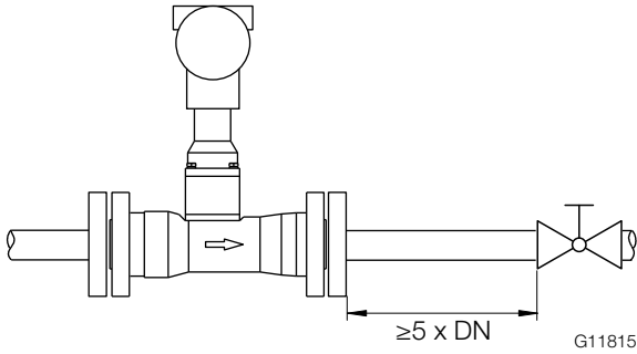
Рис. 11: Монтаж исполнительных устройств
