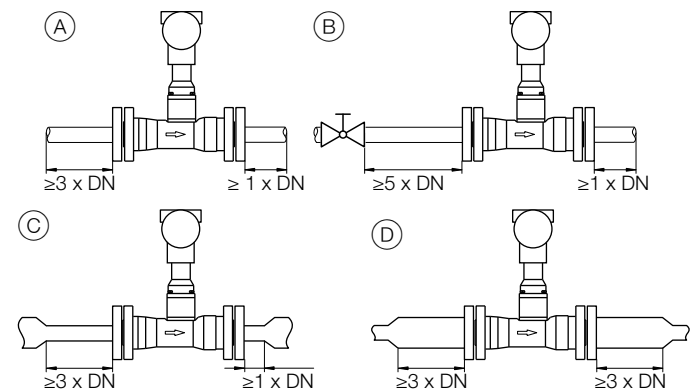
Рис. 7: Прямолинейные участки трубопровода
