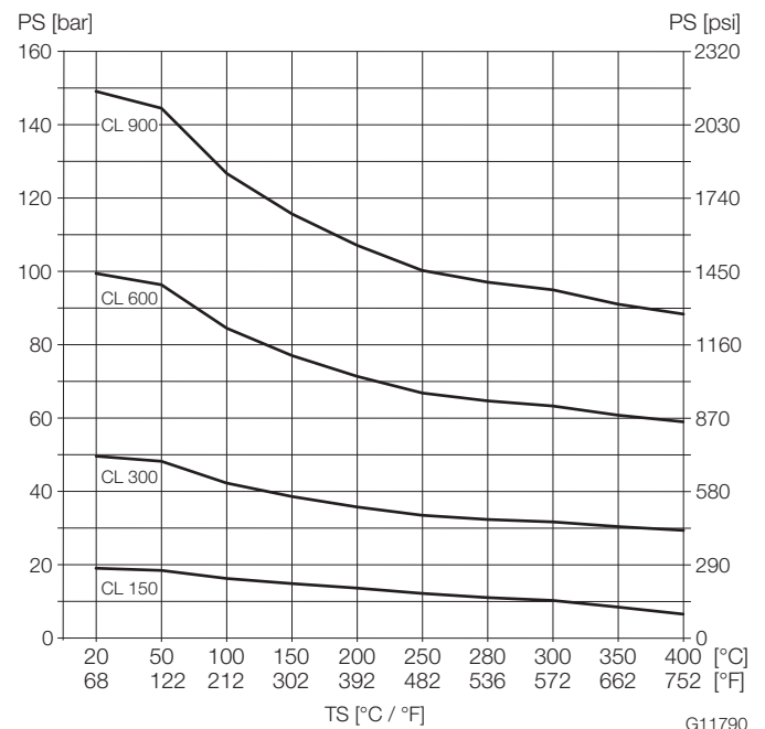
Рис. 6: Присоединительный элемент: фланец по стандарту ASME
