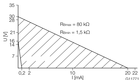
Рис. 23: Диапазон внешнего напряжения питания и тока
