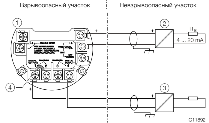
Рис. 24: Электрическое подключение (пример)
