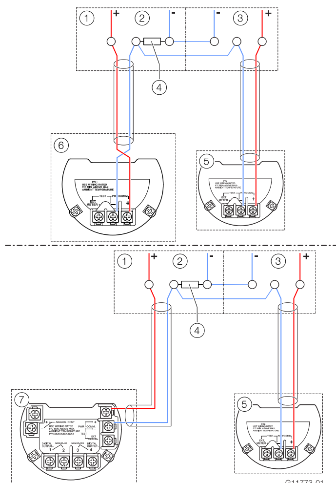
Рис. 22: Подключение измерительных преобразователей с поддержкой протокола HART (пример)
