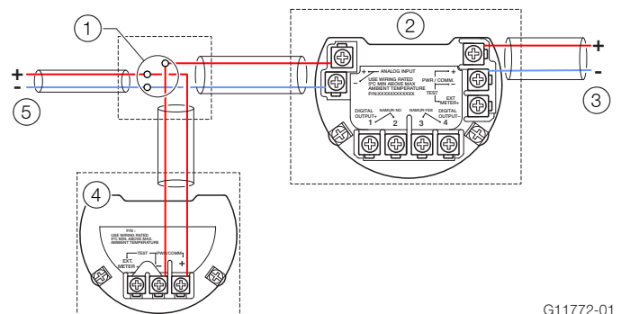
Рис. 21. Подключение измерительных преобразователей на аналоговом входе (пример)
