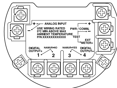
Рис. 15: Соединительные клеммы
