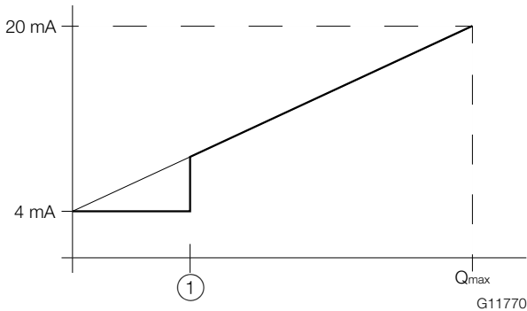
Рис. 20: Реакция, токовый выход
