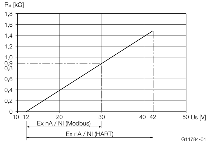
Рис. 25: электропитание в зоне 2, взрывозащита, без образования искр
