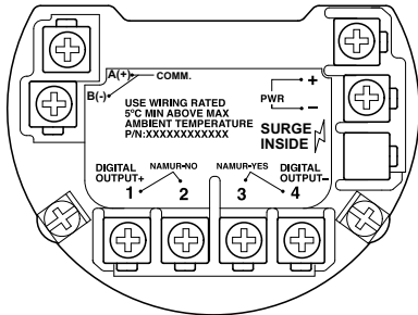
Рис. 17: Соединительные клеммы
