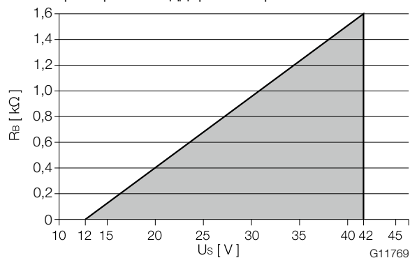
Рис. 19: Диаграмма нагрузки токового выхода; нагрузка в зависимости от напряжения питания
