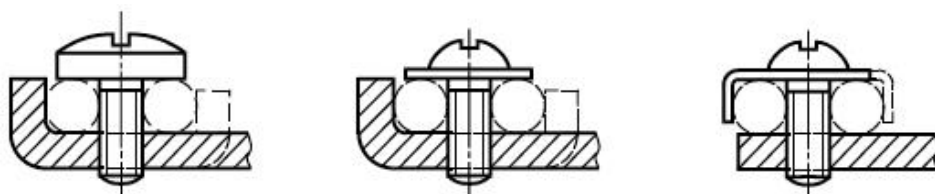
Рисунки 14b и 14с - Винтовые выводы
