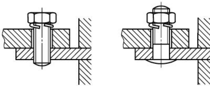
Рисунок 14ф - Выводы для шин и кабелей
