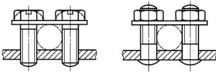
Рисунок 14е - Пластиначатые выводы
