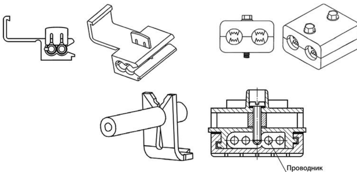
Рисунок 14i - Выводы с прокалыванием изоляции
