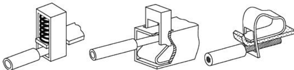
Рисунок 14h - Безвинтовые выводы
