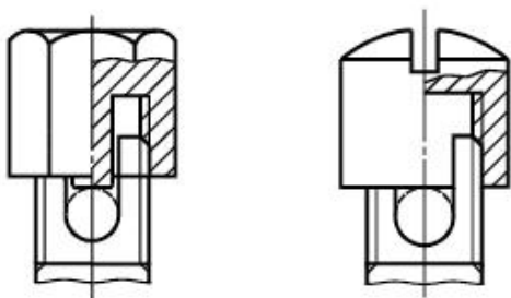
Рисунок 14г - Закрытые винтовые выводы с прижимной гайкой
