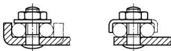
Рисунок 14d - Штыревые выводы
