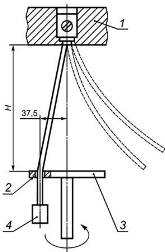
1 - фиксирующий узел; 2 - гильза; 3 - панель; 4 - груз
